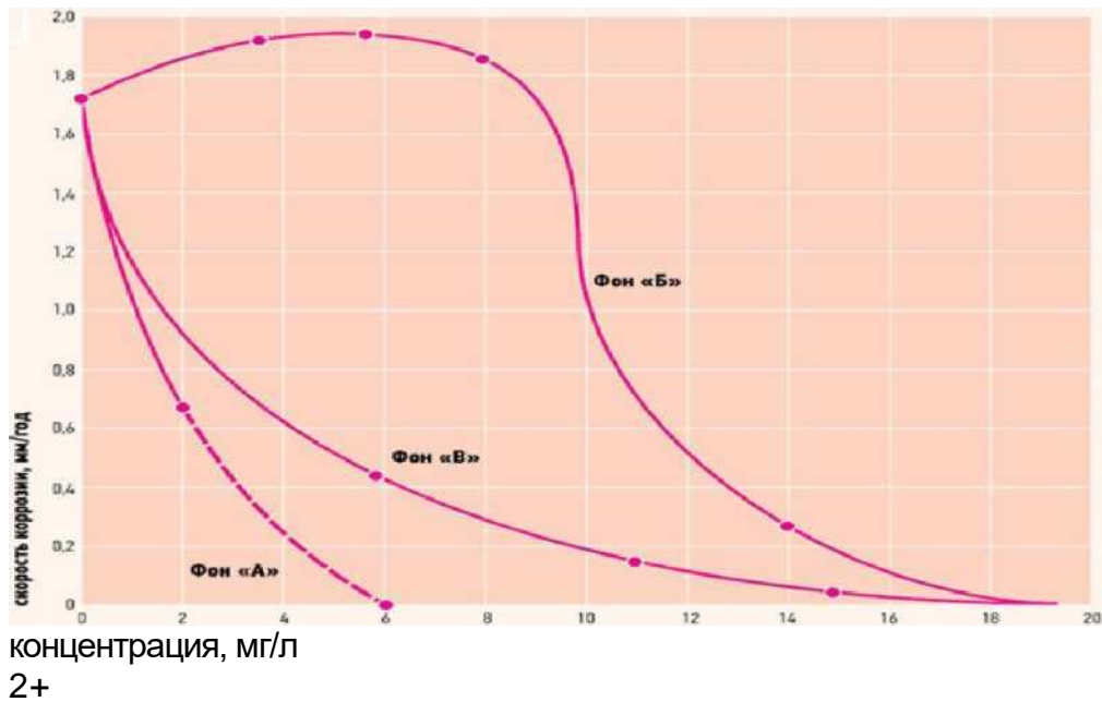
Рис.9.Изменение скорости коррозии Ст3 от концентрации ОЭДФ+Zn в медьных средах «А», «Б» и «В».
