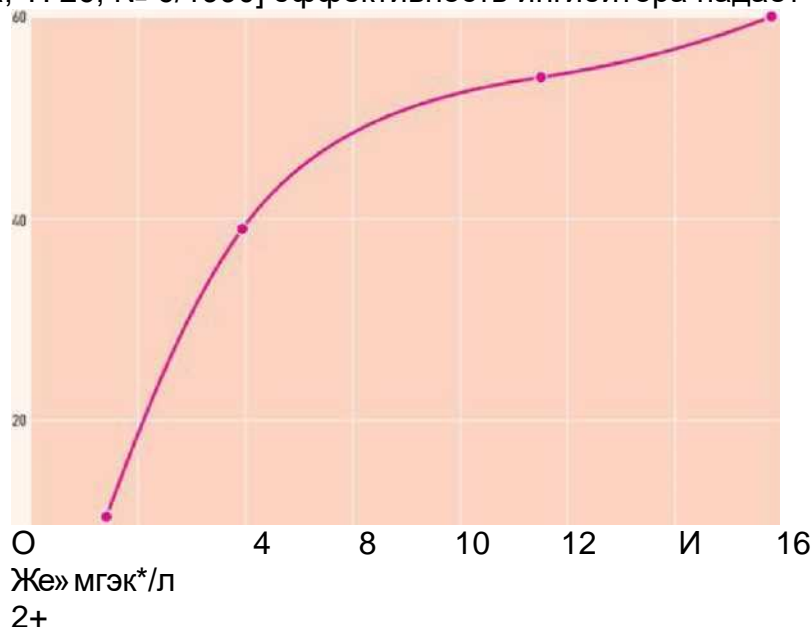
Рис.8.Зависимость потерь ОЭДФ из композиции ОЭДФ+Zn от кальциевой жесткости воды (концентрация ингибитора - 25 мг/л, pH=7,8-8,3, t=20 0 C
