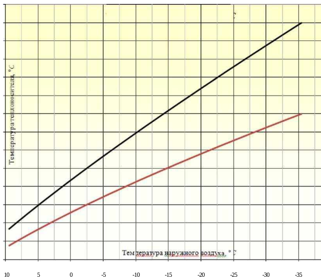
Рисунок 10. График регулирования отпуска тепла
