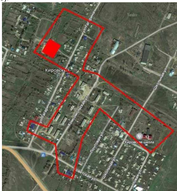
Рисунок 3. Зона действия котельной п. Кировский
