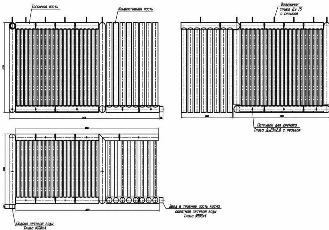
Рисунок 15. Принципиальная схема котла KBp-1,25.
